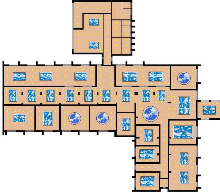
شكل (٣٠): مخطط الاسقف والانارة للدور الارضي في مركز صحي جامعة اليرموك (من عمل الباحثين)
